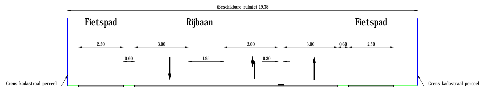
Principe dwarsprofiel A-A VRI kruispunt Schaal 1:100
